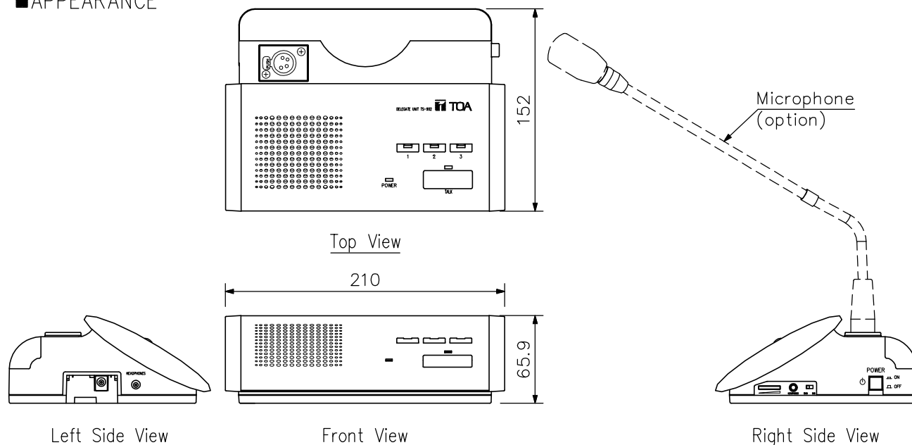
UNIT:mm SCALE:1/4
